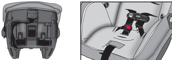
Sangle d'entrejambe dans la fente arrière
